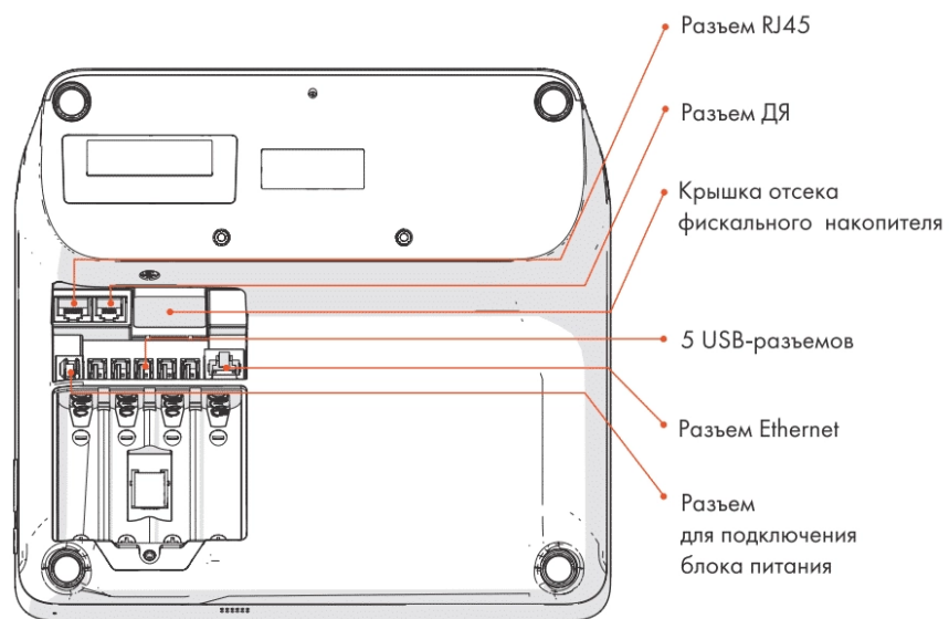
Смарт-терминал «Эвотор 10», вид снизу
